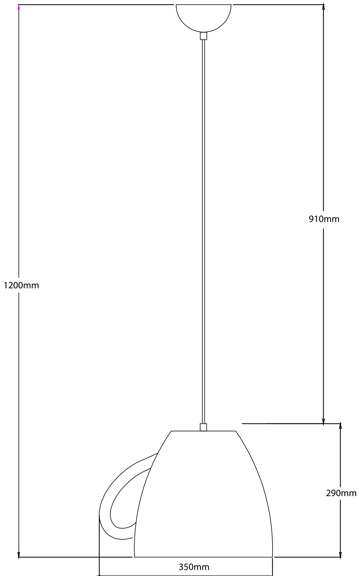
灯体尺寸: L350*W300*H1200mm
